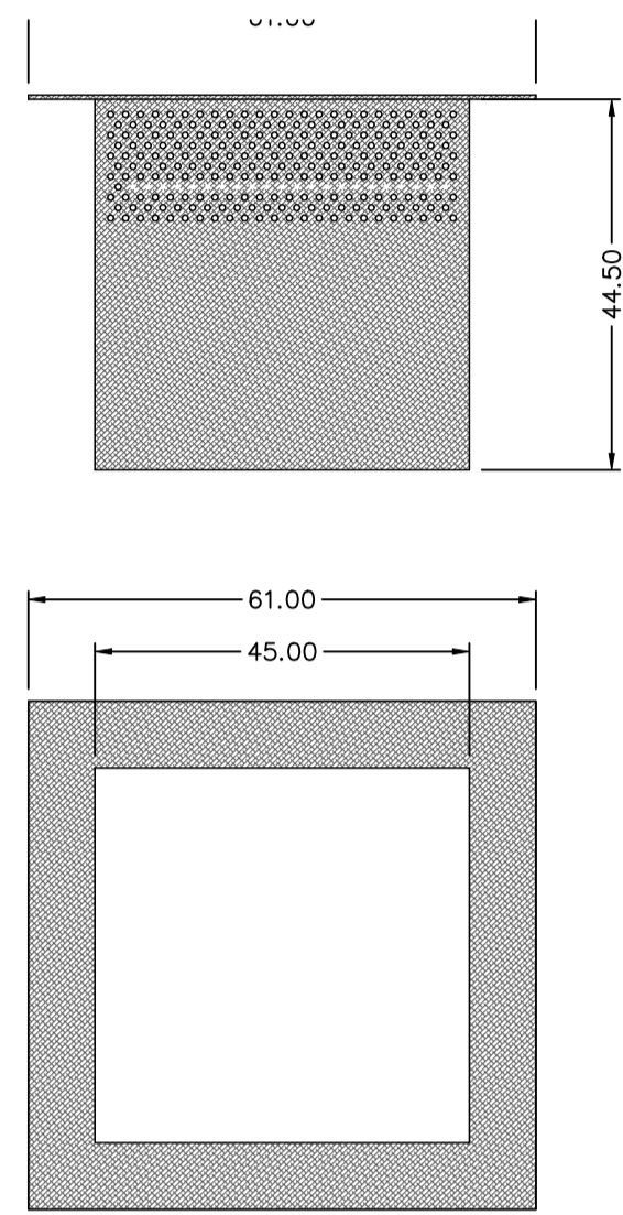
DETALLE DE ENTRADA DE PLUVIALES Y AIRE PARA PLANTACIÓN ESTOCOLMO PESO 23 Kg - ACERO INOXIDABLE Escala:1/10
