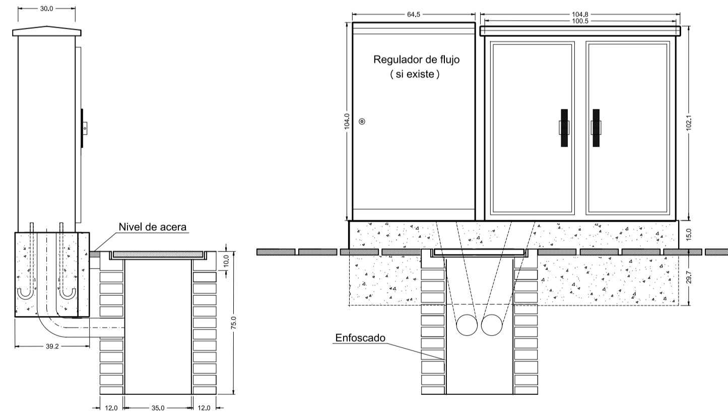
DETALLE CIMENTACIÓN CENTRO DE MANDO, PROTECCIÓN Y MEDIDA Escala 1:20
