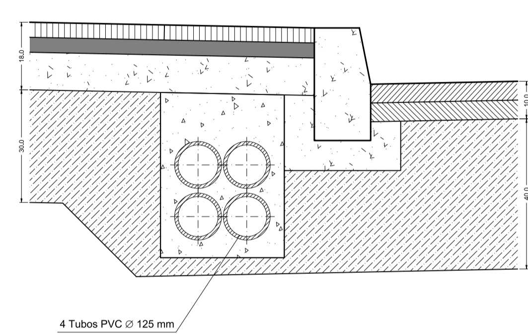
ZANJA EN ACERA Escala 1:10
