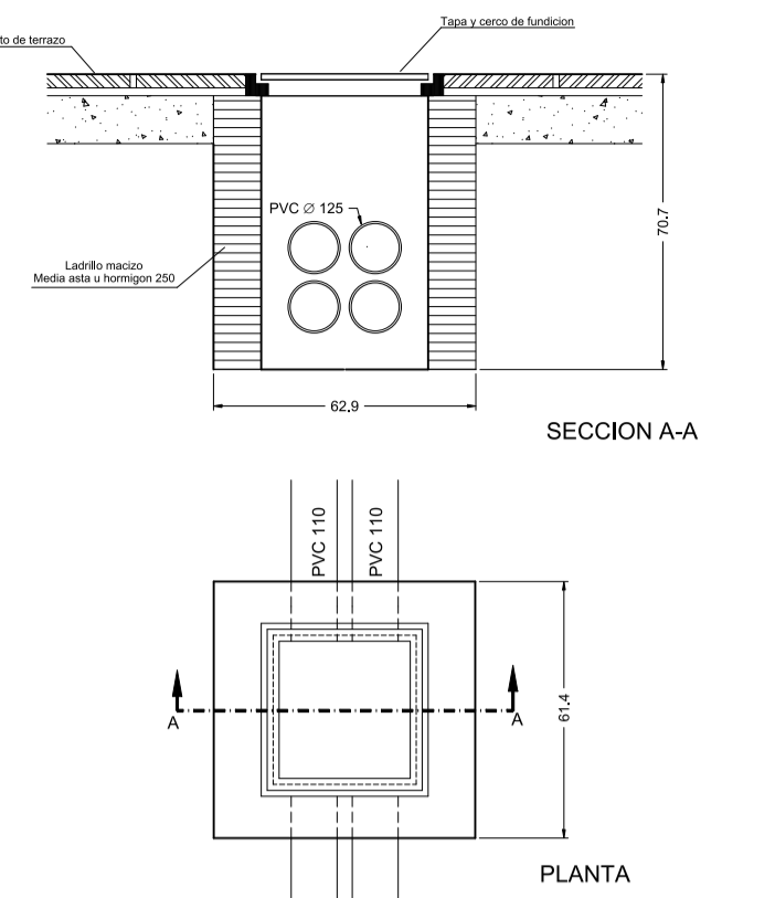
DETALLE DE ARQUETA ALUMBRADO Escala 1:20
