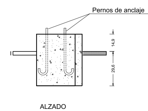
ALZADO
