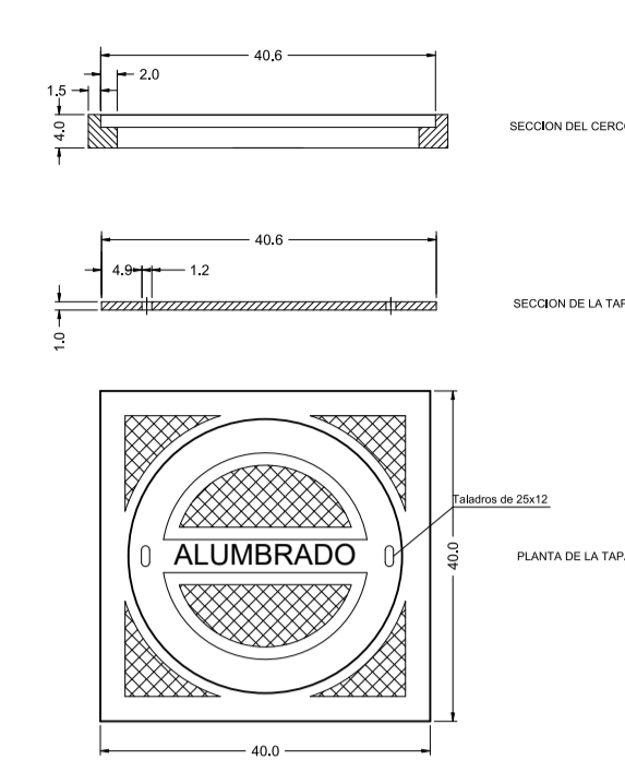
DETALLE DE TAPA Y CERCO Escala 1:10
